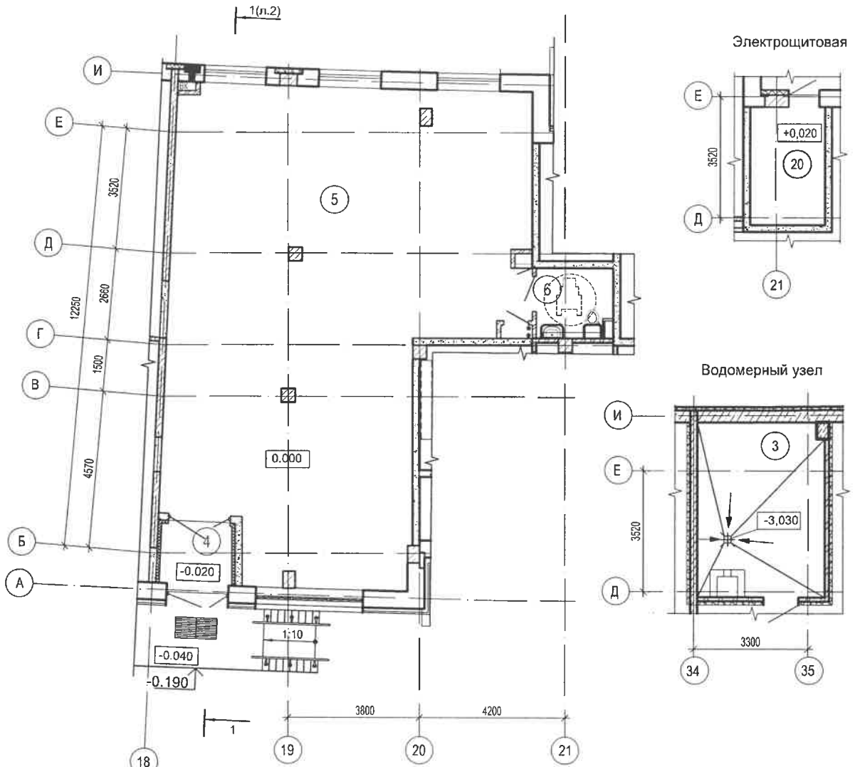
Схема здания
